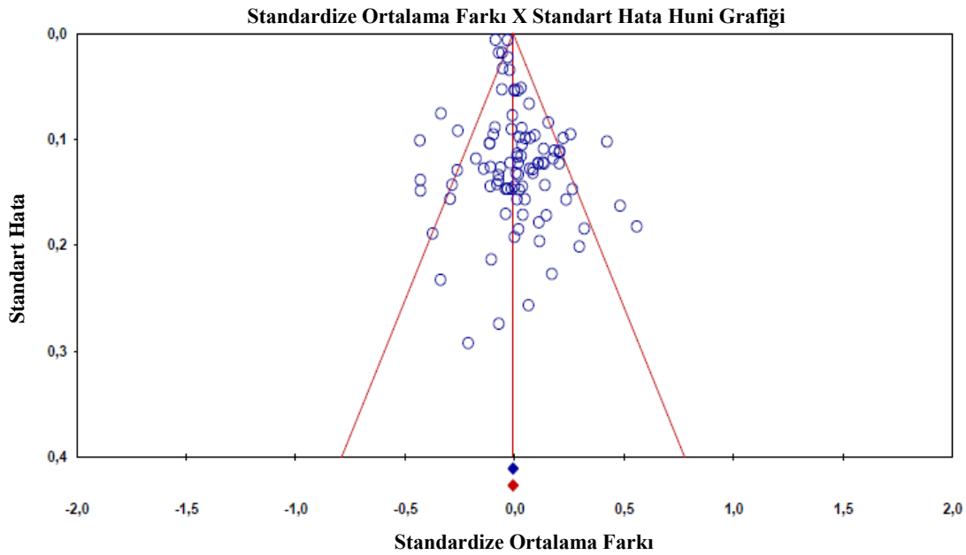
ŞEKİL 1. Yayın Yanlılığına İlişkin Huni Grafiği
